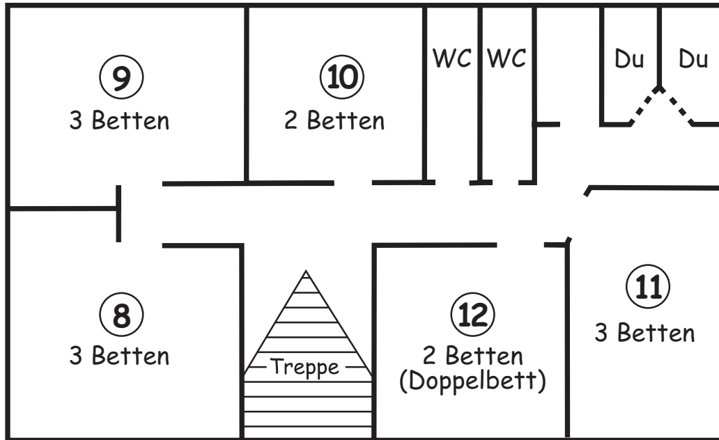
GROSSES HAUS DACHGESCHOSS
